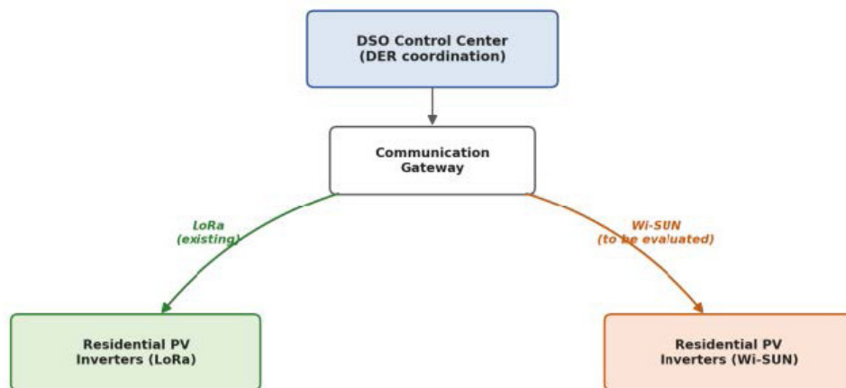
Figure 1. Architecture de communication visée entre le centre de contrôle du DSO et les onduleurs photovoltaïques résidentiels
