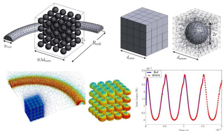
Géométries et résultats de simulations comparant les résultats de référence et ceux obtenus par homogénéisation pour un composite magnétiques doux idéalisé.
