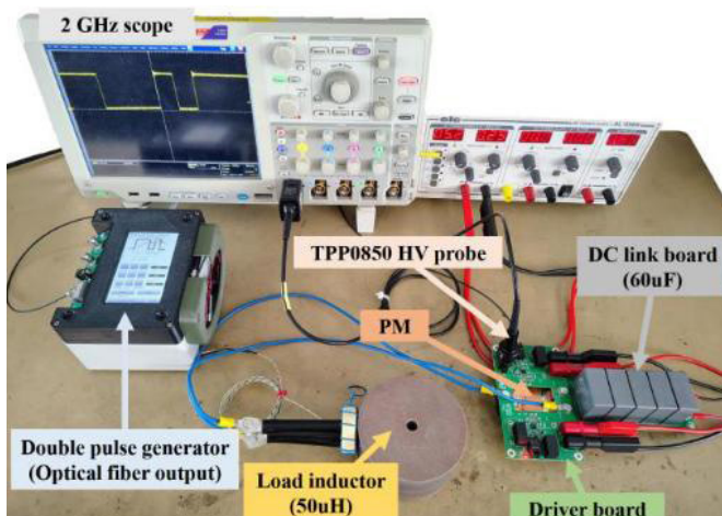
Banc expérimental mettant en oeuvre un module de puissance interconnecté avec un PCB DC link (objet du stage).
