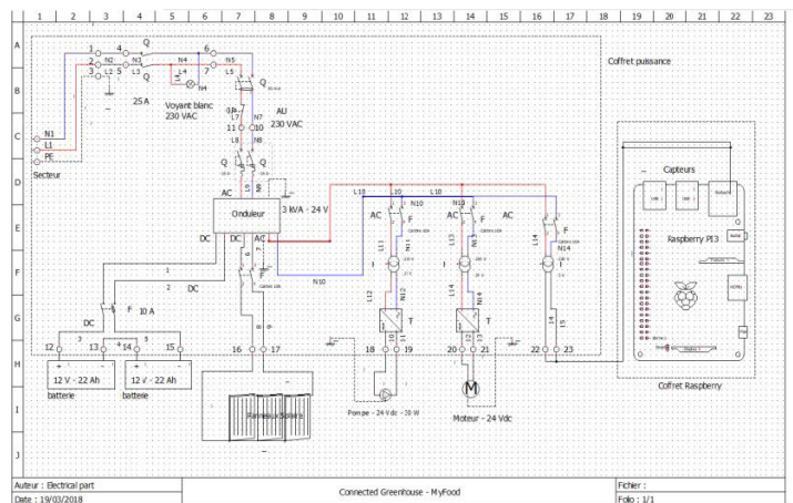
Schéma électrique de l'installation
