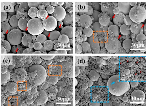
Micrographie d'un composite magnétique doux
