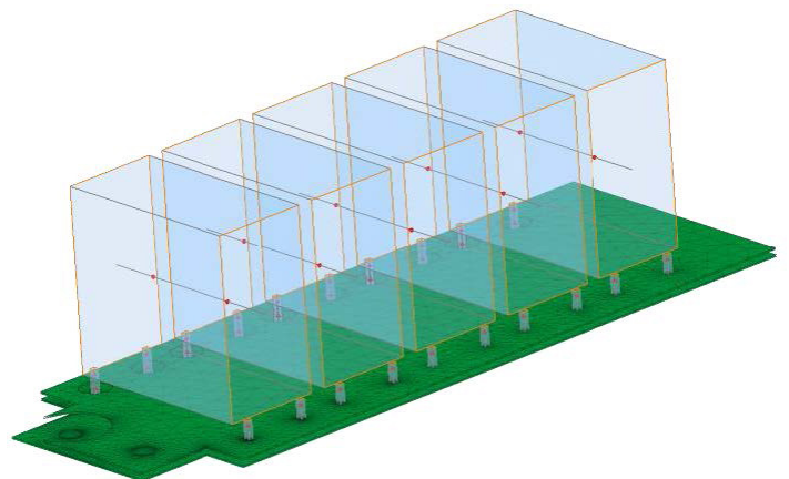
Modélisation éléments finis d'un bus DC de condensateurs sur carte PCB avec interconnexions vers le module de puissance
